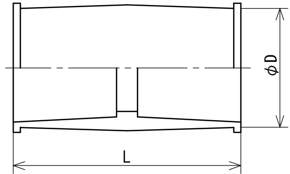
(呼び径 65 ~ 150)
